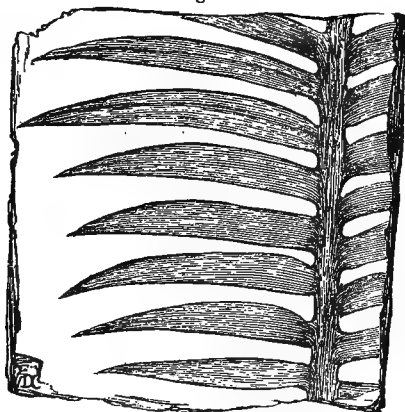
ZAMIA FENEONIS. (Portland Oolite.)
